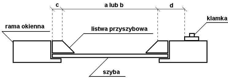
Rysunek 1: Listwa skośna
